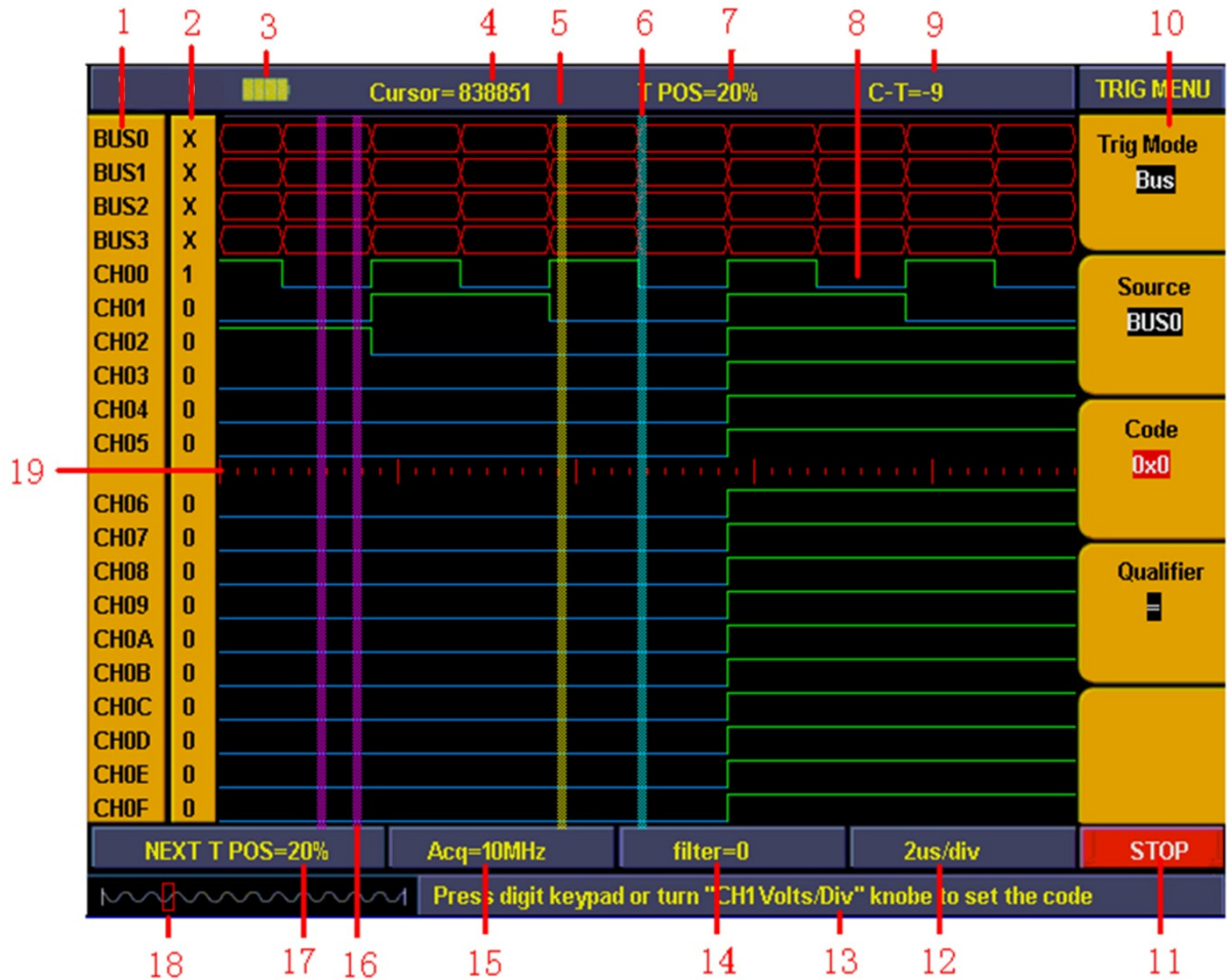
Abb. 11 Benutzeroberfläche des Logik-Analysers
