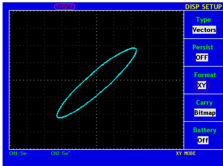
Abb. 57 Anzeigeformat XY
