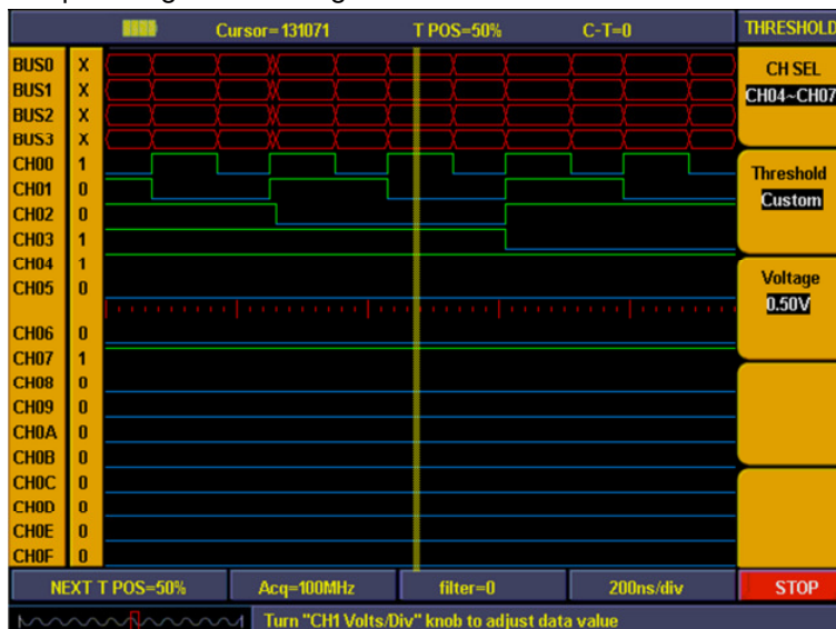
Abb. 88 Benutzerdefinierte Threshold-Einstellung
