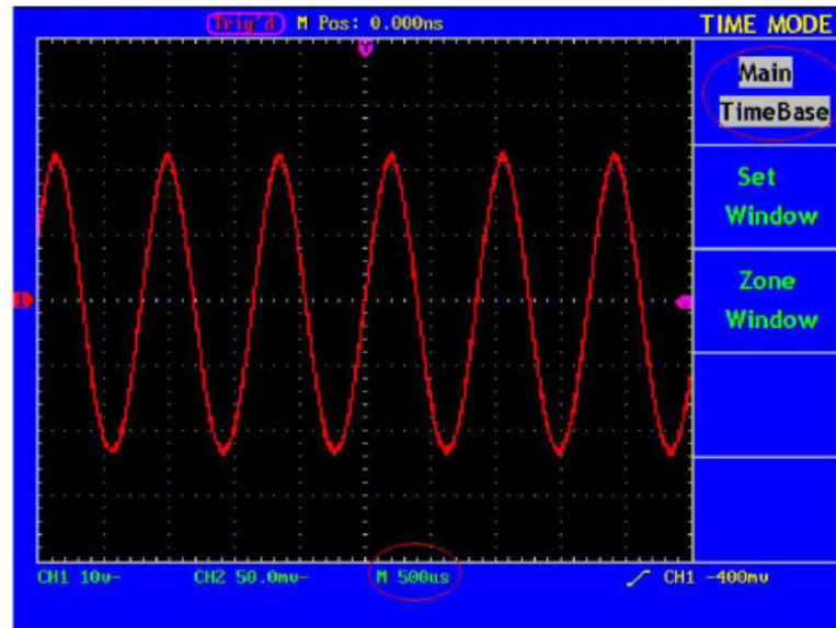
Abb. 33 Hauptzeitbasis
