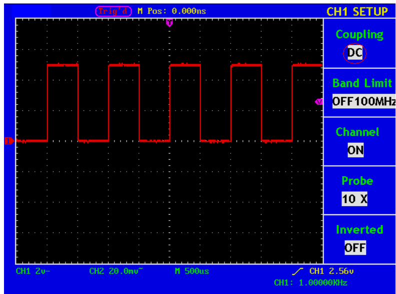
Abb. 21 DC-Kopplung Oszillogramm
