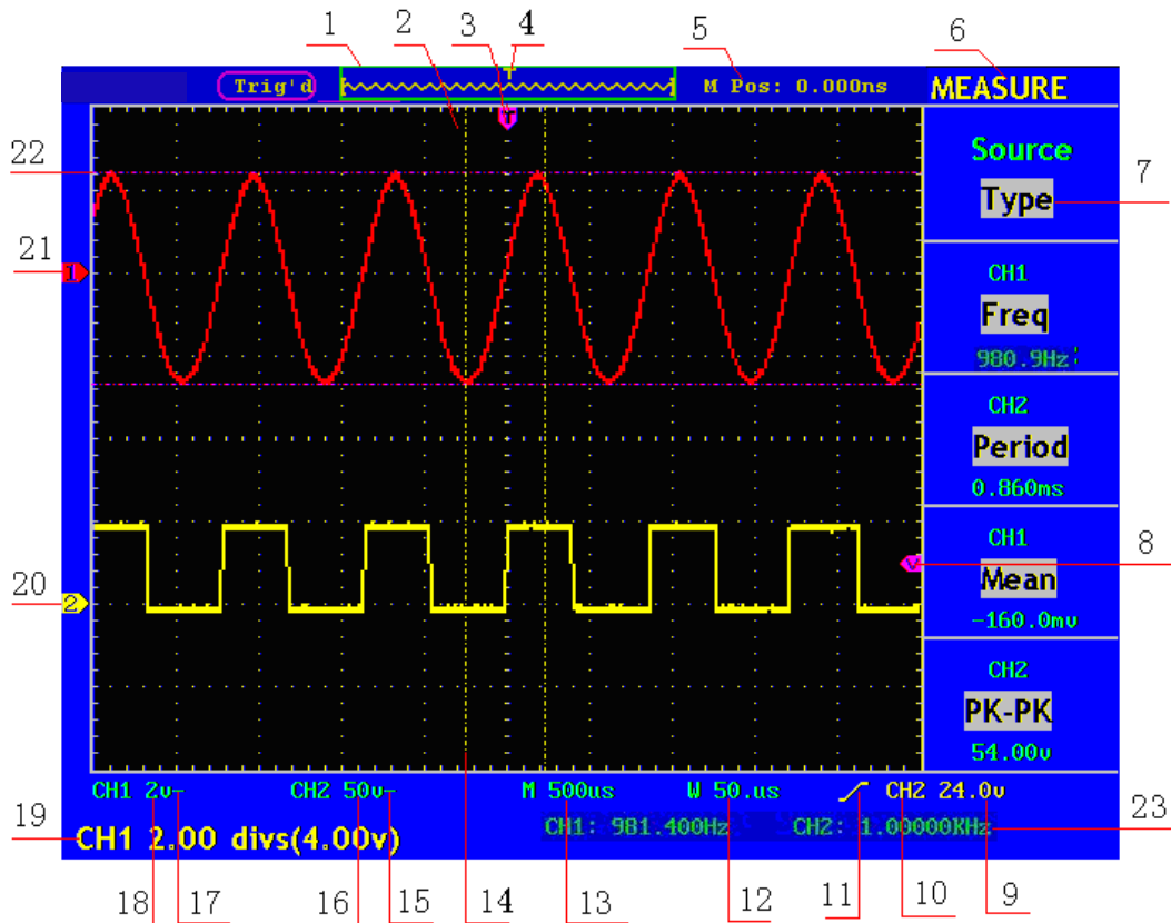
Abb. 3 Bedienoberfläche
