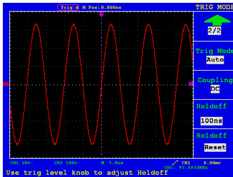
Abb. 39 Wellenform-Abstiegsflanke getriggert
