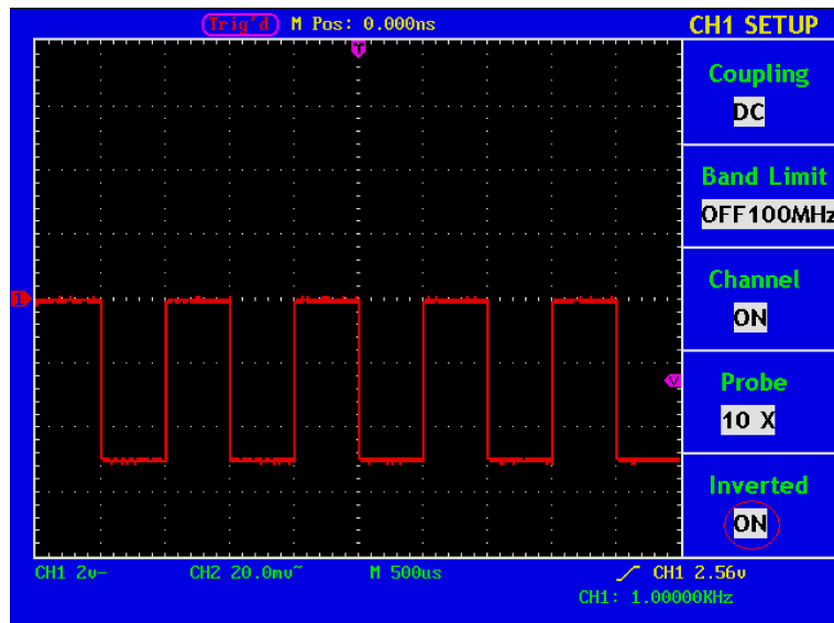
Abb. 25 Wellenform invertiert
