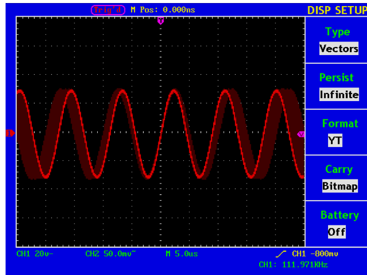
Abb. 56 Unendliche Nachleuchtzeit
