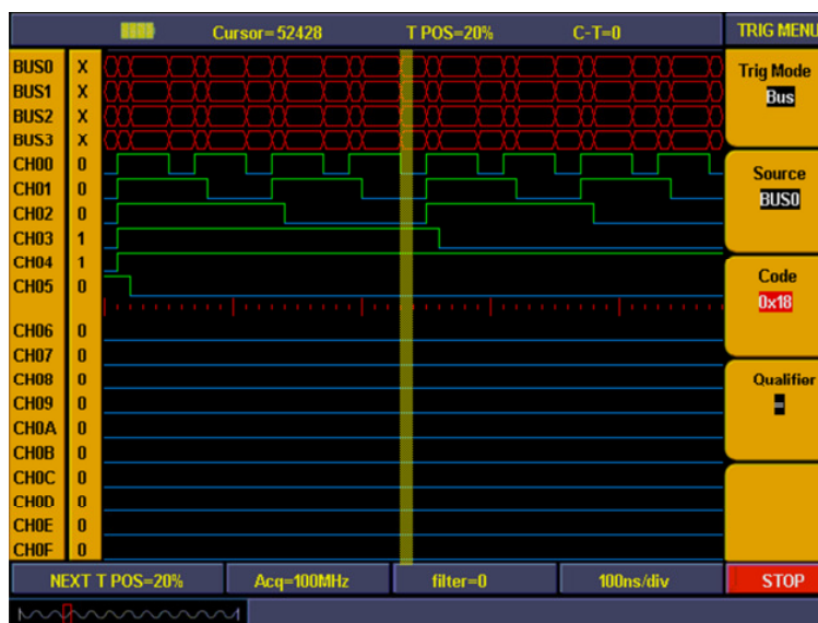
Abb. 80 Bus-Trigger
