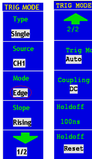
Fig. 37 Edge trigger menu
