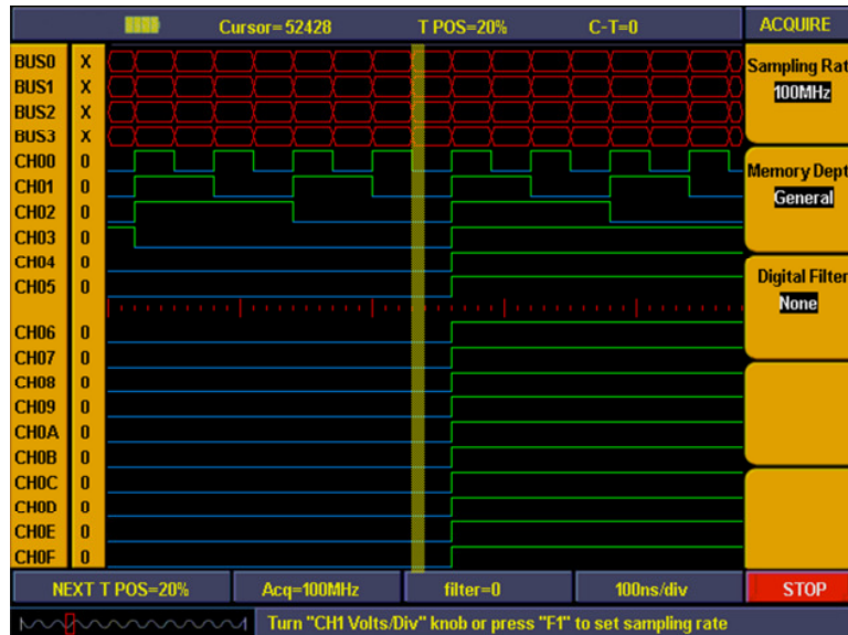
Abb. 76 Sampling-Einstellung
