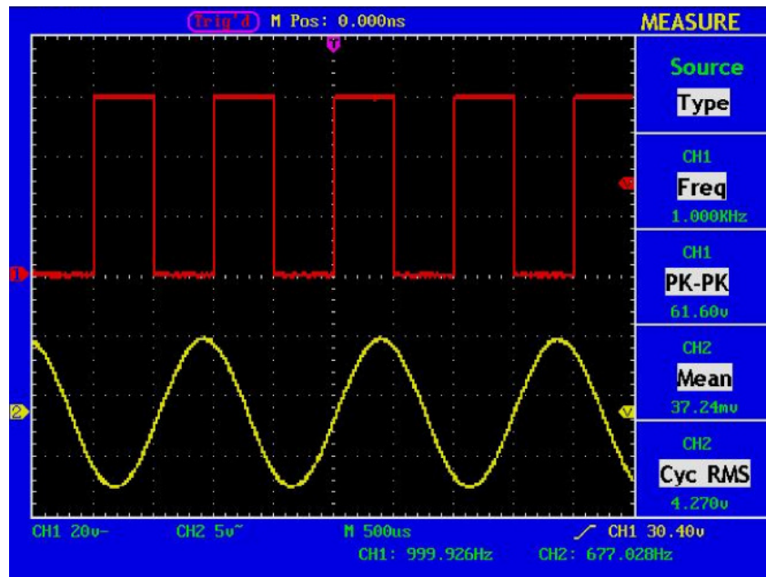
Abb. 66 automatische Messungen
