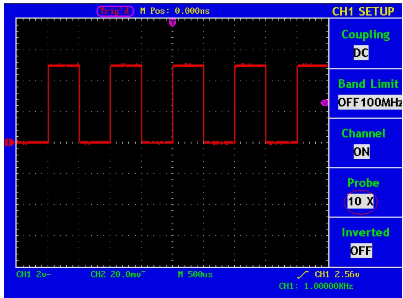
Abb. 23 Einstellen des Tastkopf-Dämpfungsfaktors
