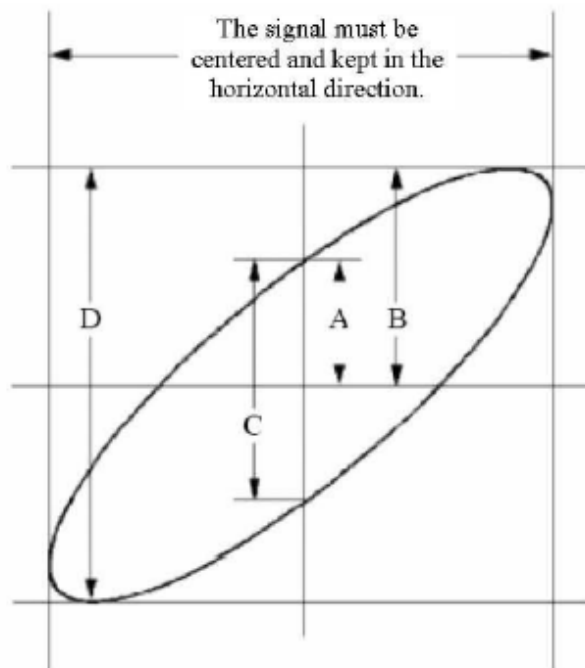
Abb. 107 Lissajousfigur
