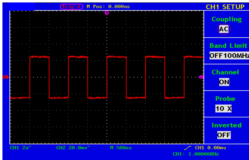
Abb. 20 AC-Kopplung Oszillogramm
